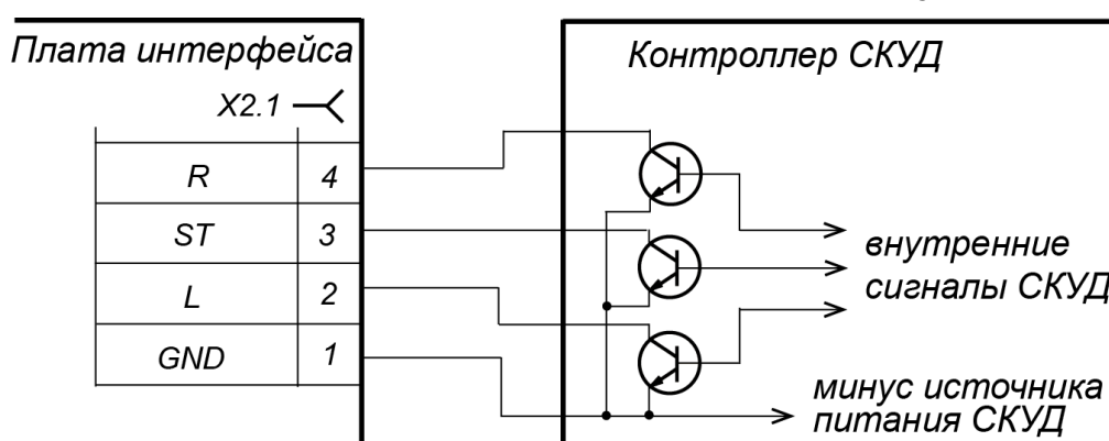
Рисунок 9. Управляющий элемент СКУД – схема с открытым коллекторным выходом
