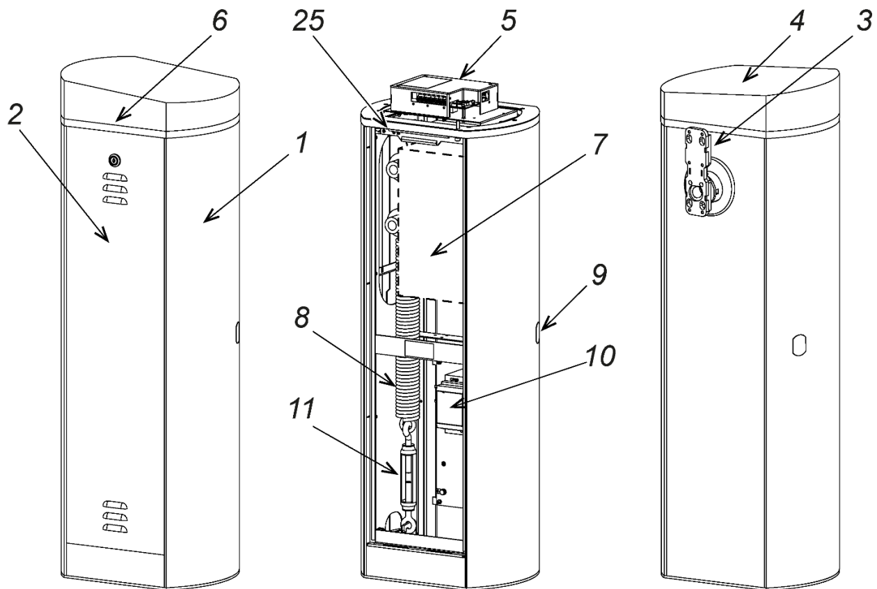
Рисунок 2. Устройство шлагбаума
