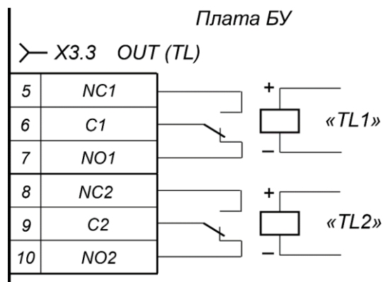
Рисунок 6. Выходные каскады для TL1, TL2
