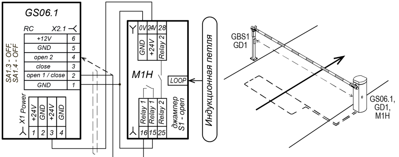
Рисунок 20. Вариант схемы подключения датчика индукционной петли для управления шлагбаумом с односторонним проездом
