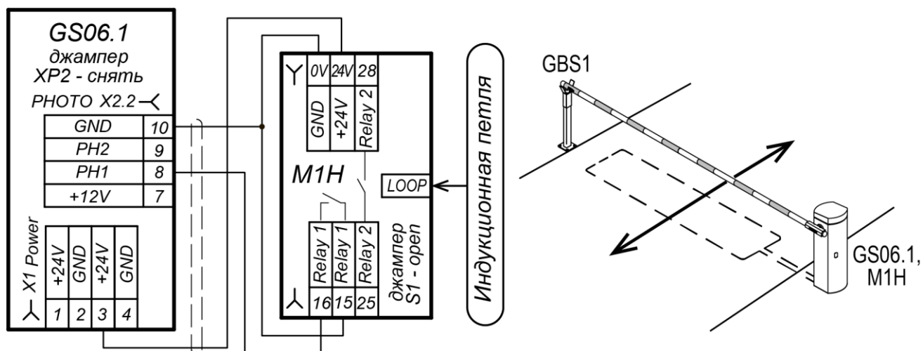
Рисунок 18. Схема подключения одноканального датчика M1H
