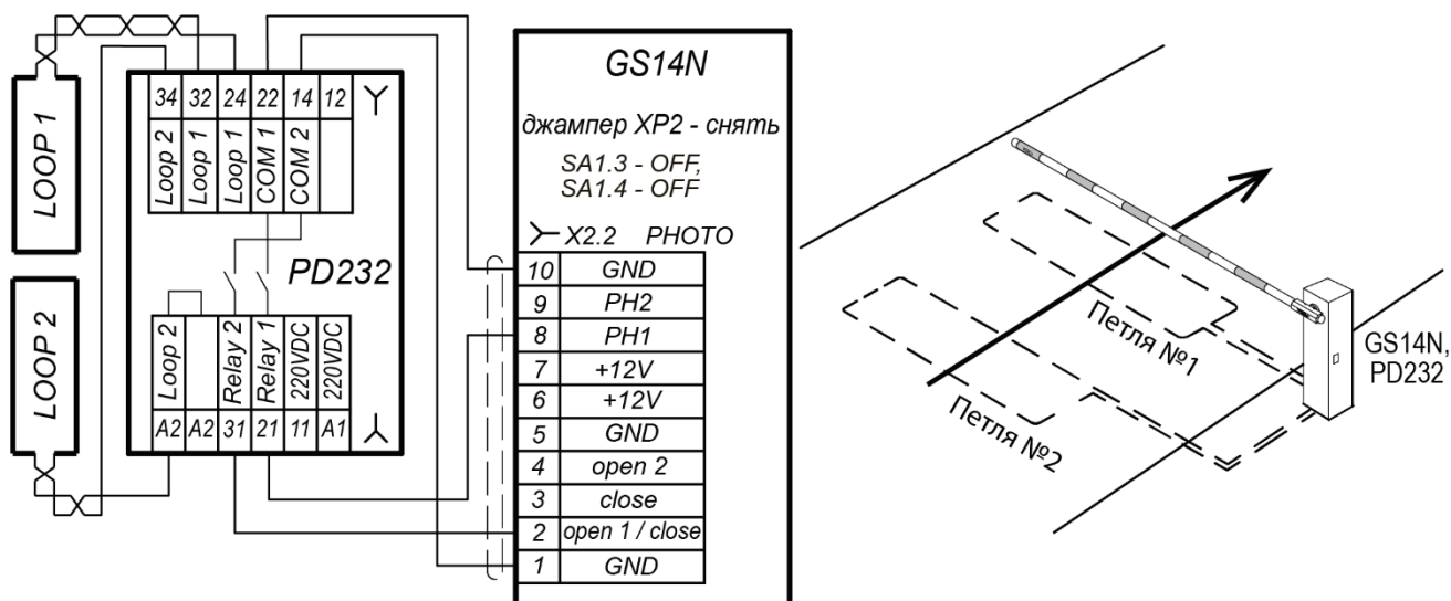
Рисунок 18. Вариант схемы подключения двухканального датчика индукционной петли для управления шлагбаумом с односторонним проездом
