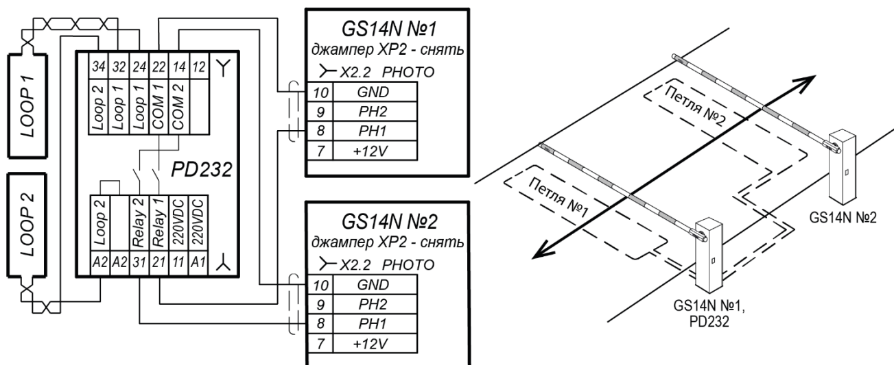
Рисунок 16. Схема подключения двухканального датчика PD232
