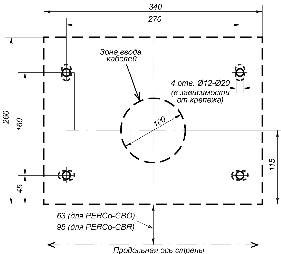
Рисунок 7. Разметка установочных отверстий шлагбаума
