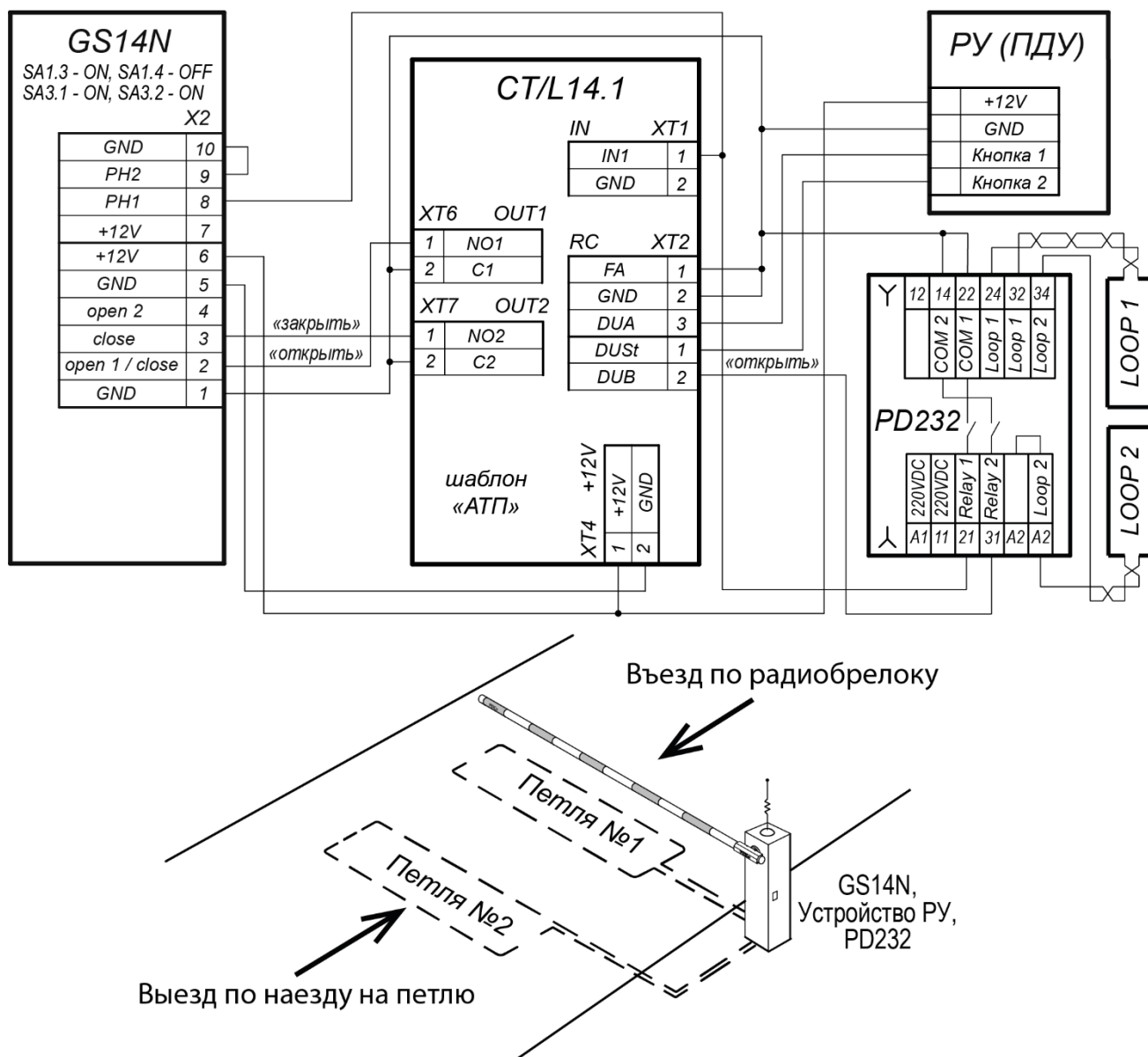
Рисунок 17. Вариант схемы подключения датчика индукционной петли для управления шлагбаумом с двусторонним проездом
