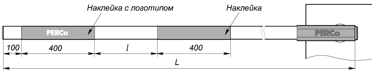
Рисунок 10. Наклеивание световозвращающих элементов на стрелу PERCo-GBR
