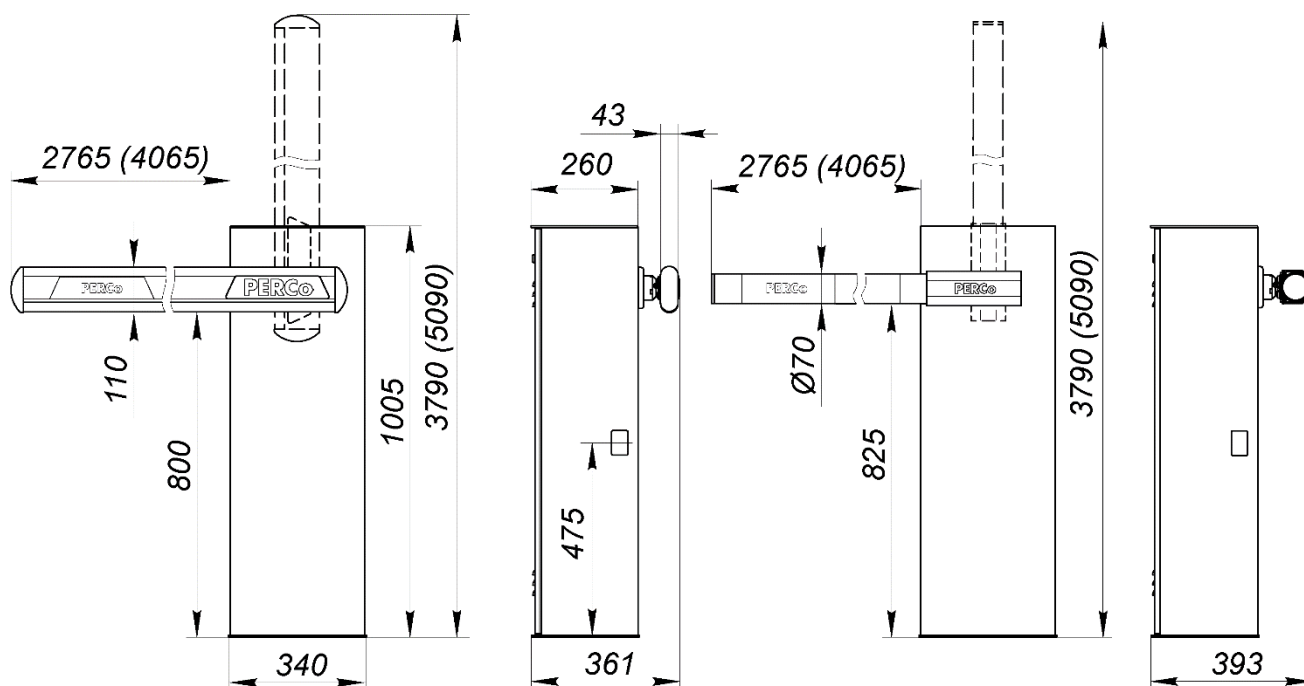
Рисунок 1. Габаритные размеры шламбаума
