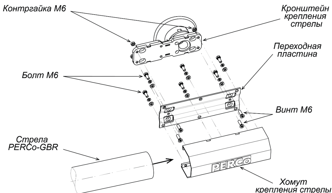
Рисунок 14. Монтаж стрелы PERCo-GBR
