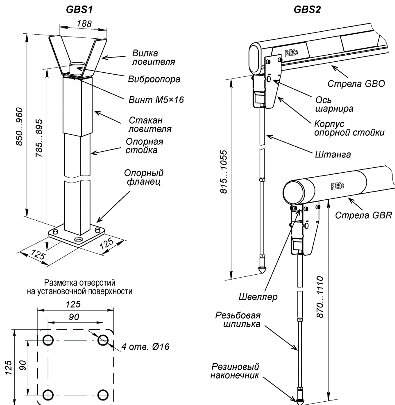
Рисунок 16. Внешний вид опорных стоек PERCo-GBS1 и PERCo-GBS2
