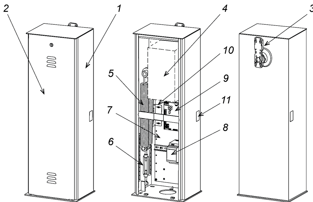
Рисунок 2. Устройство стойки шлагбаума
