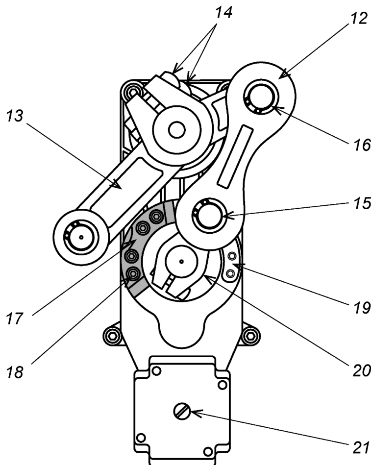
Рисунок 8. Порядок переустановки стрелы шламбаума
