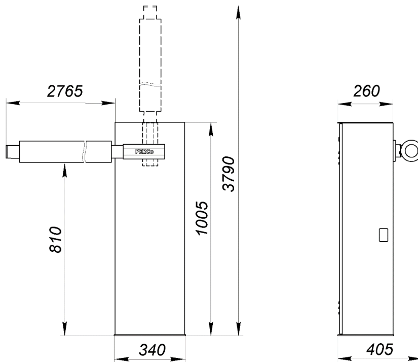
Рисунок 1. Габаритные размеры шлагбаума
