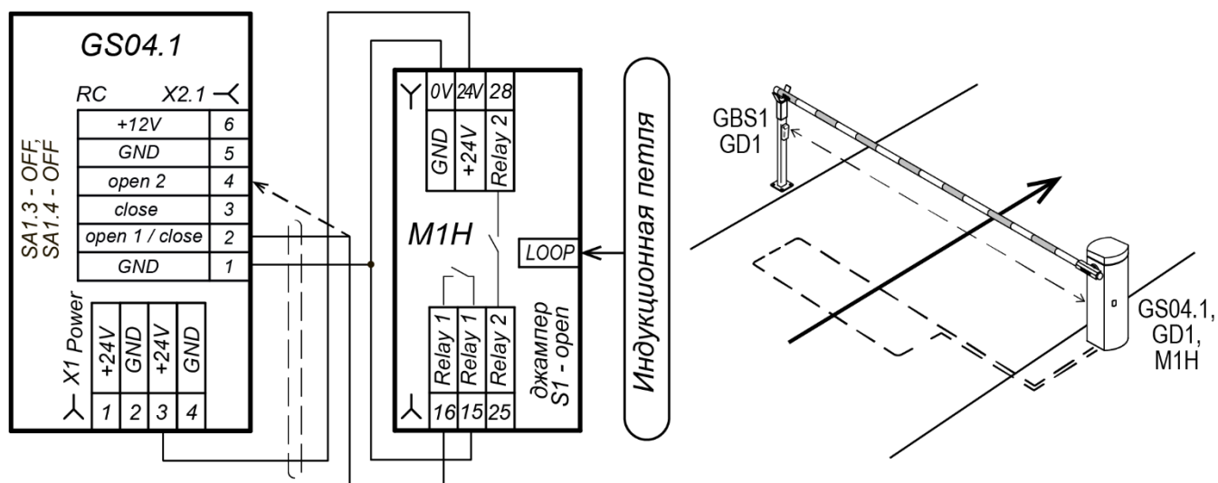
Рисунок 23. Вариант схемы подключения датчика индукционной петли для управления шлагбаумом с односторонним проездом
