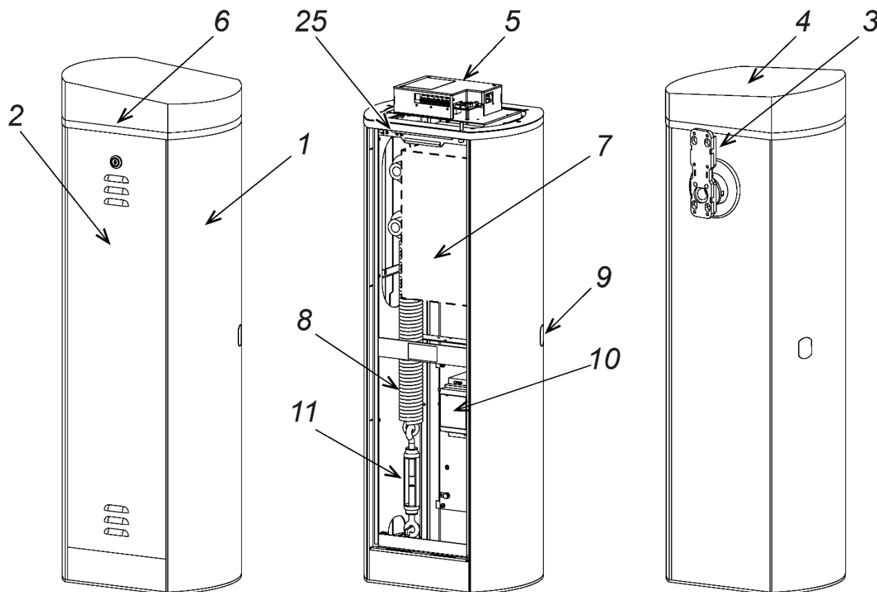
Рисунок 2. Устройство шламбаума
