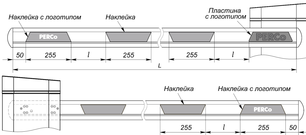
Рисунок 13. Наклеивание световозвращающих элементов на стрелу PERCo-GBO
